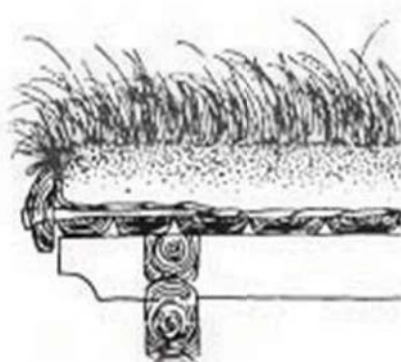
Фронтон с ветровой доской. Берёзовая кора уложена с напуском на доску
